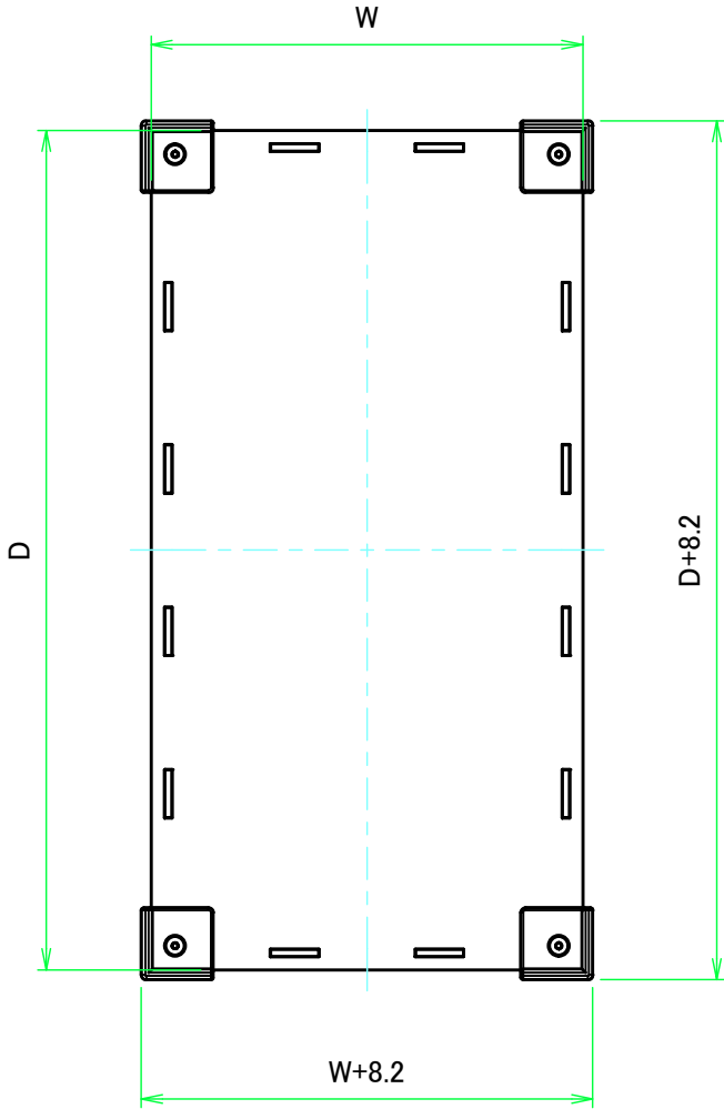
Wパネル1 / W Panel 1
