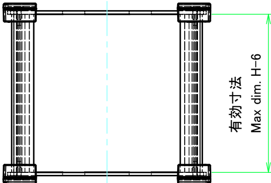
Wパネル1 / W Panel 1
